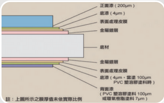
註：上圖所示之膜厚值未依實際比例
